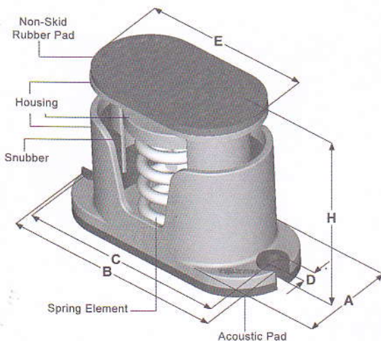
PTM-CG, PTM-CG2
